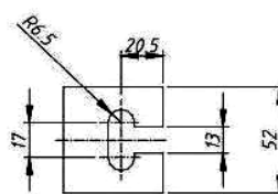
吊掛架詳細尺寸
