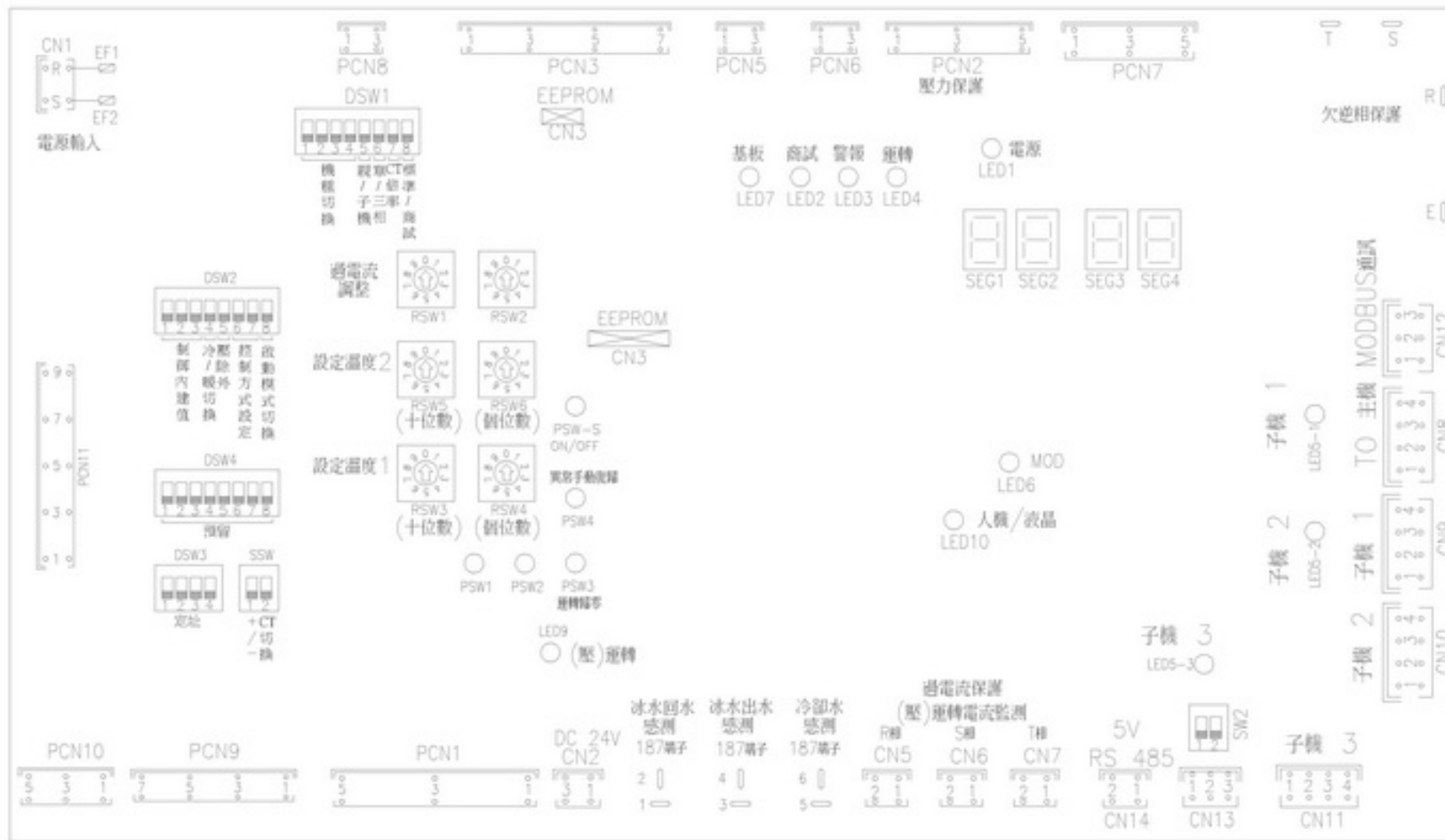
圖6-2 基板外觀圖
