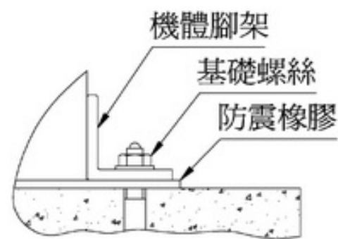
圖 4-3 基礎構造示意圖
