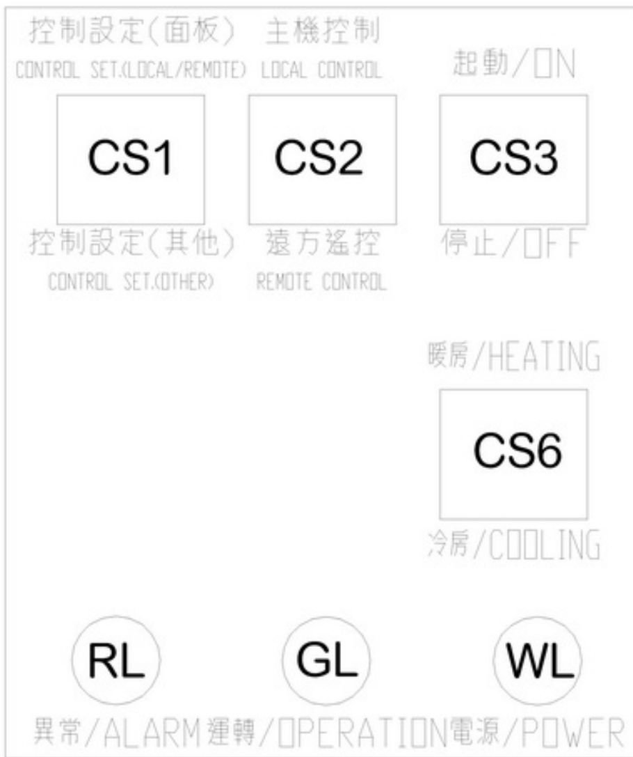
操作面板配置圖
