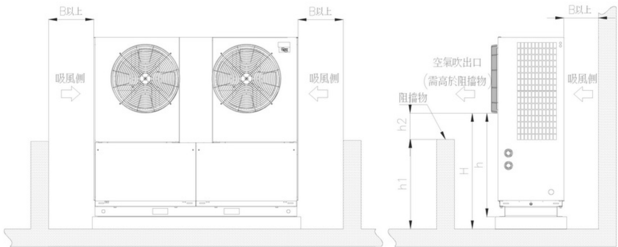
圖 4-1 安裝場所示意圖
