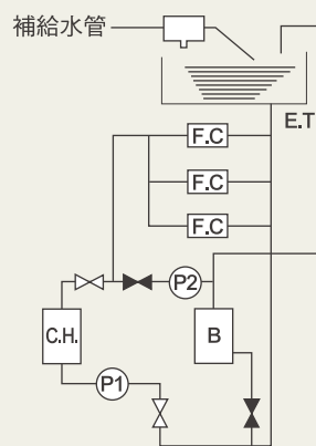
<冰水機配管圖例>
