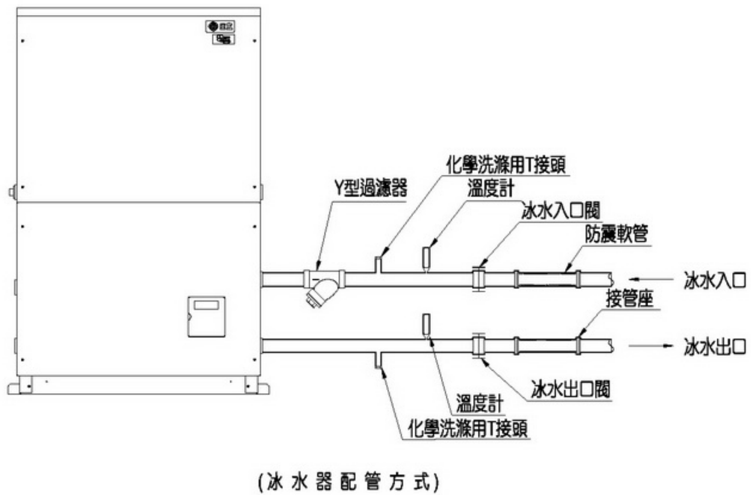
圖 4-5 水配管施工要領 (Y型過濾器限RCU-N81、101W機種使用)
