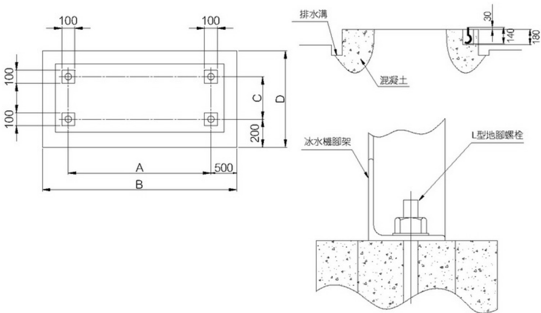
圖 4-2 安裝基礎示意圖
