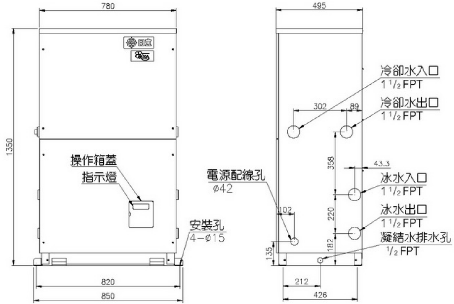
內部結構圖
