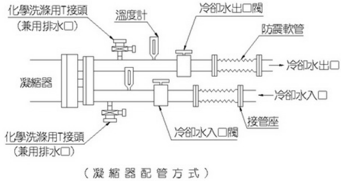
圖 4-4 水配管施工要領
