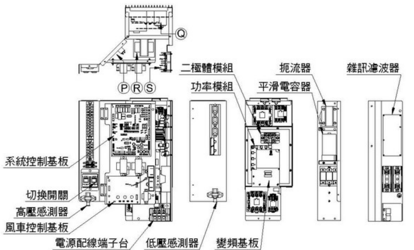
電氣板詳圖 P方向視圖 Q方向視圖 R方向視圖 S方向視圖
